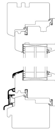
POIKKILEIKKAUS, PUUKARMI
