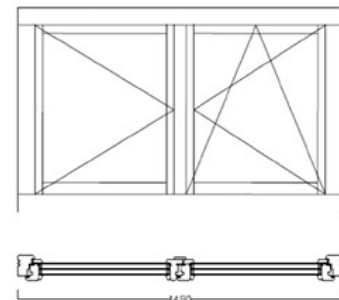
DK-IKKUNAN PERIAATEKUVA, B-MALLI, KOHTAAVILLA PUITTEILLA
