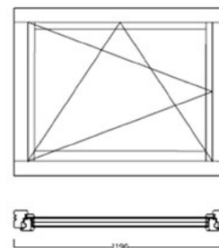
DK-IKKUNAN PERIAATEKUVA, A-MALLI
