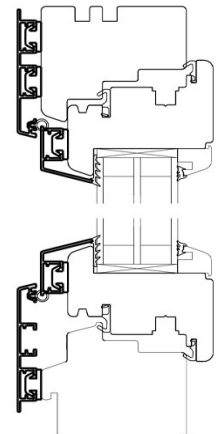
POIKKILEIKKAUS, ALUMIINIKARMI
