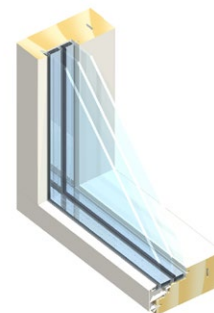
MEK U-value 3K: 0,80, 2K: 1,3
